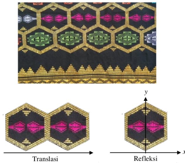
Gambar 3. Transformasi geometri pada motif subahnale
