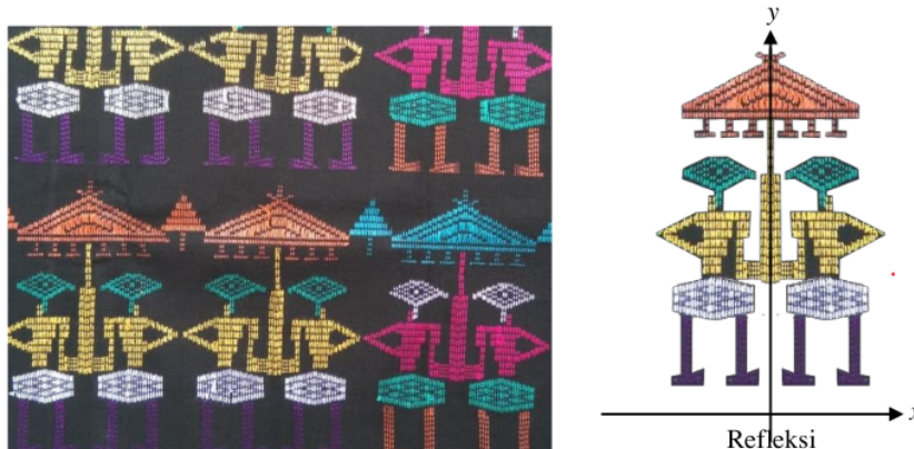
Gambar 2. Transformasi geometri pada motif wayang
