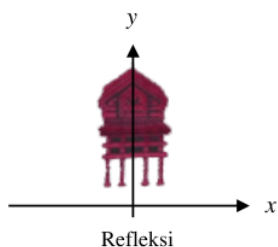
Gambar 6. Transformasi geometri pada motif alang/lumbung
