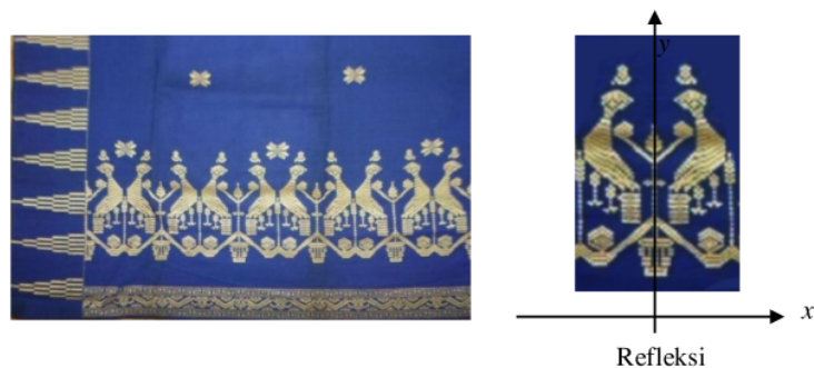
Gambar 4. Transformasi geometri pada motif keker
