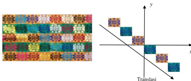
Gambar 5. Transformasi geometri pada motif bintang empat
