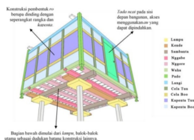
Gambar 6. Konstruksi Ro Uma Jampo Sumber: (Falaqie Chandra No Hikari, 2017)
