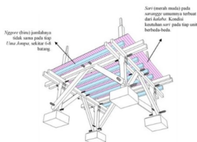
Gambar 4. Konstruksi Sarangge Uma Jampo Sumber (Falaqie Chandra No Hikari, 2017)
